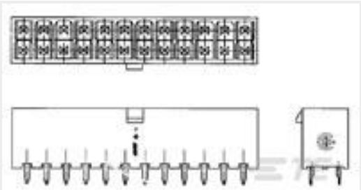
TE 产品编号2-1586038-2 22P VRT HDR VAL-U-LOK V0
