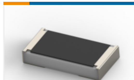
TE 产品编号6-2176231-1 SMD 功率电阻器 : 3 瓦特 , 1% Tol
