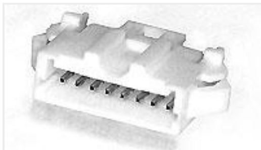
TE 产品编号 1-292230-3 1.5 MINI CT SGL V SMT W/BOSS 1
