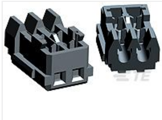
TE 产品编号 6-353293-9 MINI CT MT REC ASSY 19P BLUR
