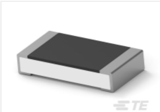
TE 产品编号5-2176387-2 RQ 1206 453K 0.1% 10PPM 1K RL
