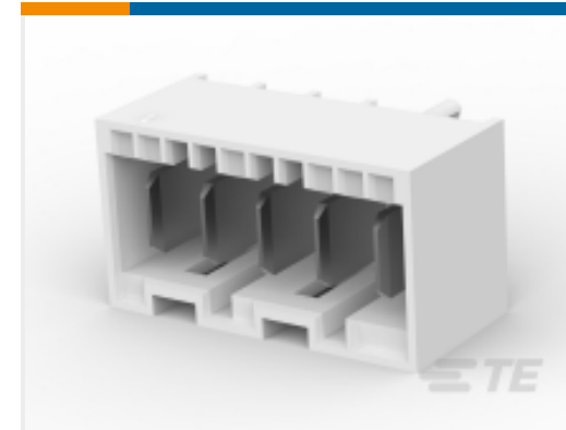
TE 产品编号 1-1971895-5 5P, RAST 5 Tab Header, THV
