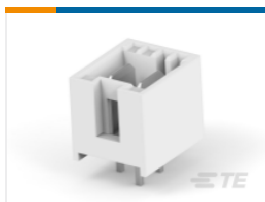
TE 产品编号 4-1971895-2 2P, RAST 5 Tab Header, THV
