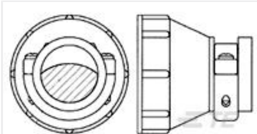
TE 产品编号182663-1 13 SIZE CPC STD CLAMP
