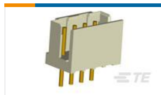
TE 产品编号 6-292165-3 CT P/HDR BOX V 3P T/P BLACK
