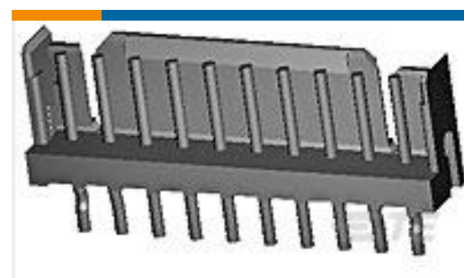
TE 产品编号 6-292170-3 CT P/HDR ASSY 3P V W/O KINK T
