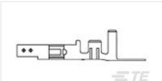
TE 产品编号794958-2 VAL-U-LOK SKT BR AU 22-26AWG
