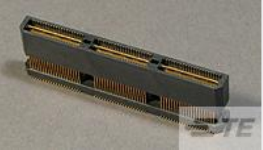
TE 产品编号 1658048-3 MSB0.80PL19ASY120FL,-,F,-TY
