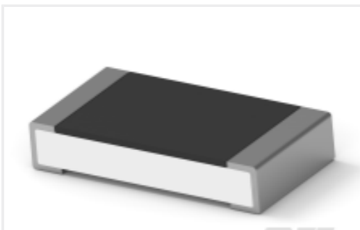
TE 产品编号1-2176391-0 RQ 1206 15K4 0.1% 10PPM 5K RL
