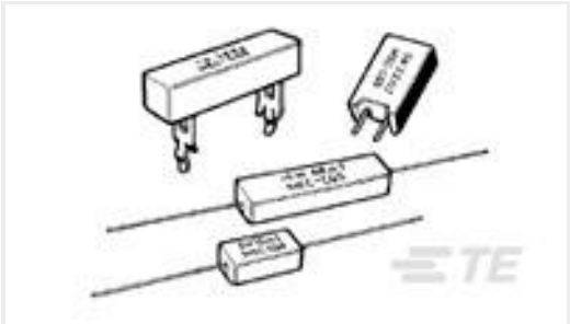
TE 产品编号6-1623795-8 SQP10 390R 5% WIRE
