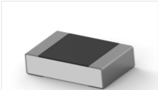
TE 产品编号2-2176374-7 RQ 0805 200R 0.1% 10PPM 1K RL
