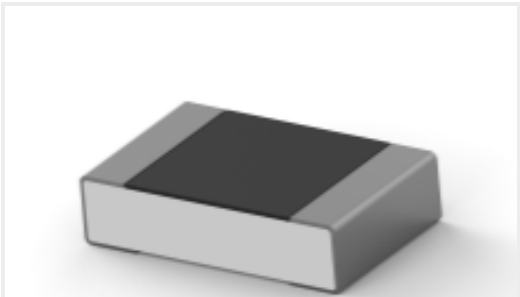
TE 产品编号8-2176374-2 RQ 0805 750R 0.1% 10PPM 1K RL
