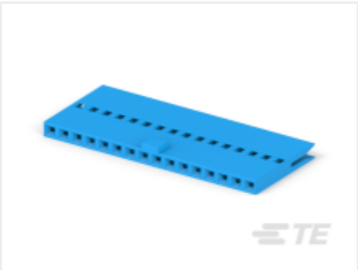
TE 产品编号CAT-F439-S01339254 2.54mm FFC 连接器母端子
