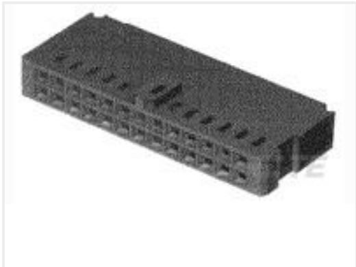
TE 产品编号1-102387-0 50 MODIV HSG COMP DR .100 POL
