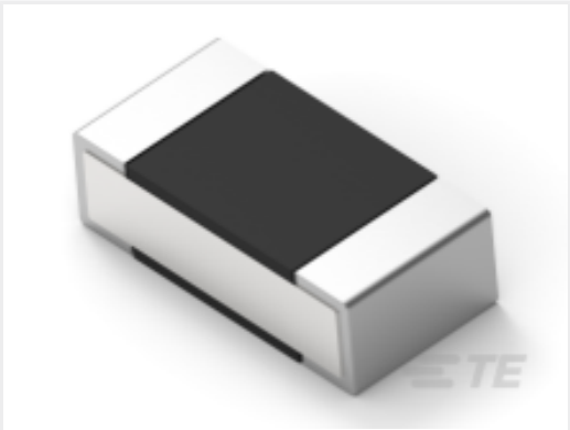
TE 产品编号9-2176310-0 RP 1E 0.1W 909R 0.1% 25PPM 1K RL
