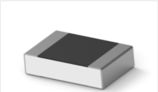
TE 产品编号7-2176379-8 RQ 0805 681R 0.1% 10PPM 5K RL
