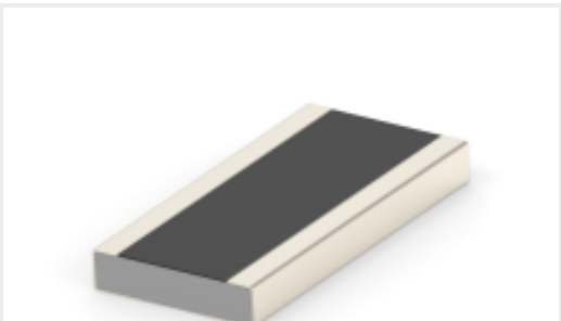
TE 产品编号1-2176545-3 RLW73P H2 1% R10 200ppm 4k RL
