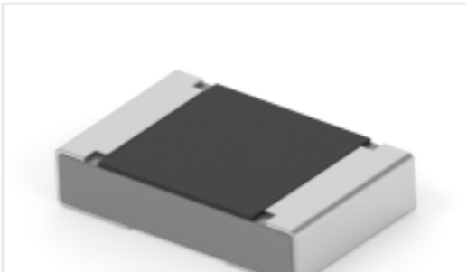
TE 产品编号4-2176478-7 RA73F 2A 17K8 0.1% 1K RL
