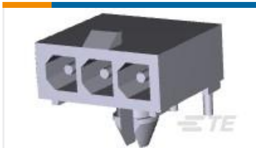
TE 产品编号1-770967-0 03P MINI UMNL R/A HDR ASSY SN
