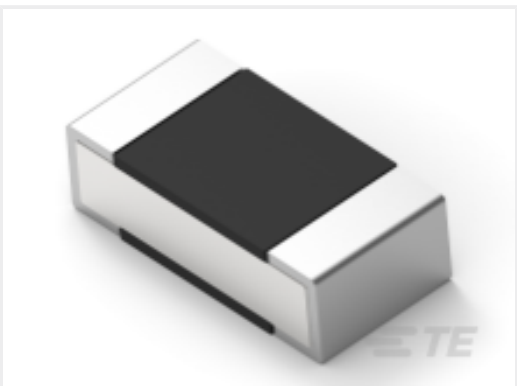
TE 产品编号6-2176304-1 RP 1E 0.1W 42R2 0.1% 25PPM 5K RL
