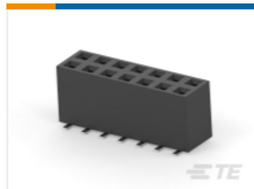
TE 产品编号1-2271630-4 MODU2.54 REC 14P DRST SMT FG MH 7.5
