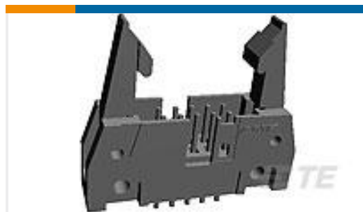
TE 产品编号5499910-2 A/L UNIV HDR 14P VERT SHT LAT
