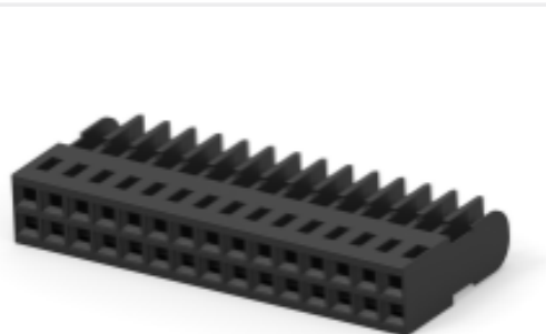
TE 产品编号 1-102394-3 30 AMP MODU MT HSG DR .100CL
