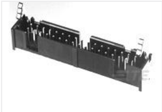
TE 产品编号2-1761608-6 IDC LOW PRO HDR 16P VERT SHT L
