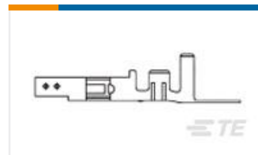
TE 产品编号 794958-1 VAL-U-LOK SKT BR SN 22-26AWG
