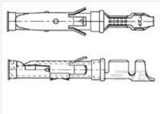
TE 产品编号163084-1 RECEPTACLE
