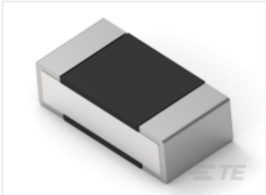
TE 产品编号9-2176312-1 RP 1E 0.1W 107K 0.1% 25PPM 1K RL
