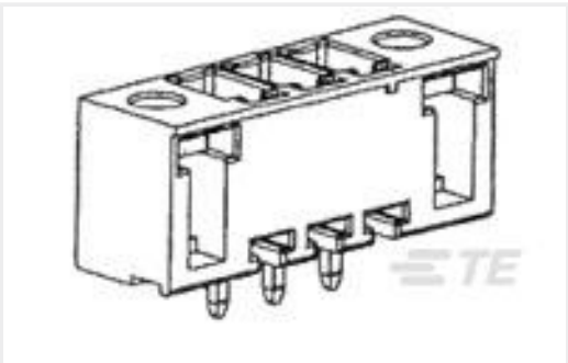
TE 产品编号796867-9 9 POS TERMI-BLOK HDR VERTICAL
