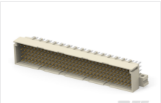
TE 产品编号384294-E STVE 160 M ABCDE VVVV 4-00 GA06 3,9 * 2
