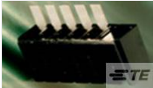
TE 产品编号 5146800-1 BATT INT,KEYLESS,5P,7.2V
