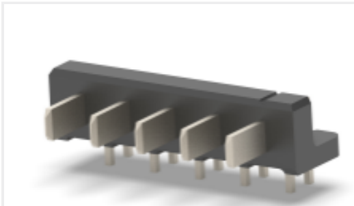
TE 产品编号 5787441-1 HDR ASY,RA,NO KEY,STR TAIL
