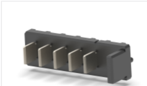
TE 产品编号 5787421-1 HDR ASY,VERT,RET TAIL,10.8V
