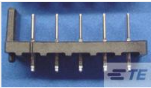
TE 产品编号 5787419-1 HDR ASY,VERT,STR TAIL,10.8V
