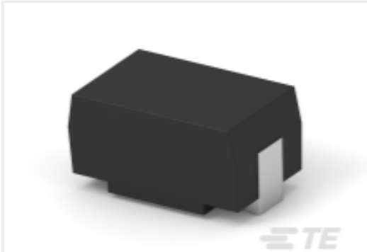
TE 产品编号CAT-C339-SM1 SMD 功率电阻器：7 瓦特，200-2M 欧姆
