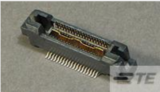
TE 产品编号 5767111-8 MICT,PLG,038,ASY,.025 TAPE CAP
