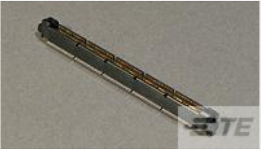
TE 产品编号 1-5767118-2 MICT,PLG,190,ASY,.025,TAPE PKG
