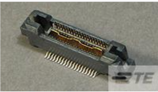
TE 产品编号 5767119-8 MICT,PLG,038,ASY,.025,TAPE PKG
