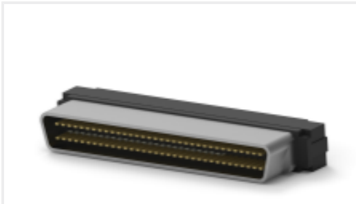
TE 产品编号CAT-AM7-22507 IDC D-Sub：连接器套件，插头，信号，1.27mm
