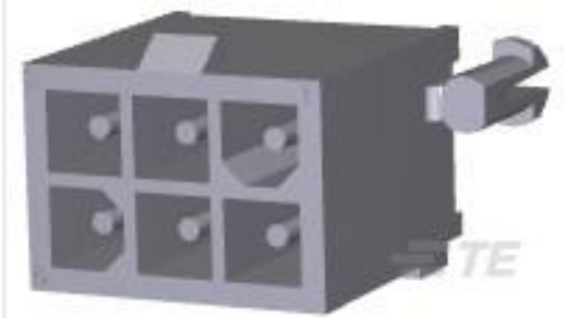
TE 产品编号1-770875-1 06P MINI UMNL HDR ASSY AU LF
