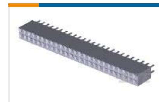
TE 产品编号2-534206-5 50 MODII VRT DR CE 100/115
