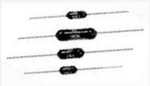
TE 产品编号6-1879663-5 H8 499R 0.1% 15PPM
