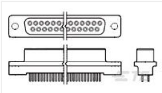
TE 产品编号5745077-6 HD-20 RCPT 15P VERT FFSCRLK
