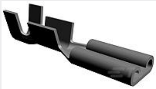
TE 产品编号61454-1 WRAP TYPE TAB RECEPTACLE 24-20 AWG TPBR
