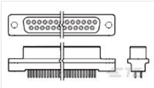
TE 产品编号5745078-6 HD-20 RCPT 25P VERT FFSCRLK
