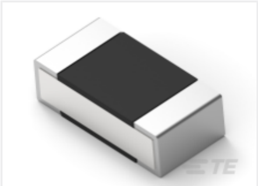
TE 产品编号8-2176307-2 RP 1E 0.1W 86K6 0.1% 25PPM 5K RL
