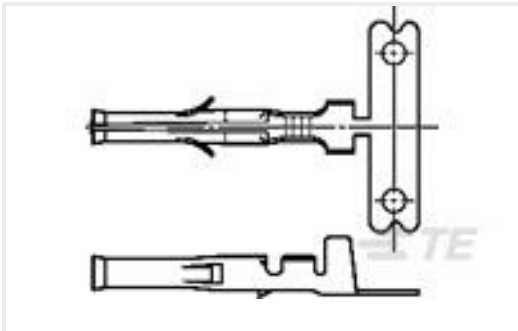
TE 产品编号350628-1 .062 COMM P&S SOK 18-24 PTPBR
