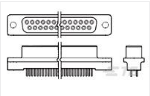
TE 产品编号5745057-4 HD-20 RCPT 15P VERT THD INS
