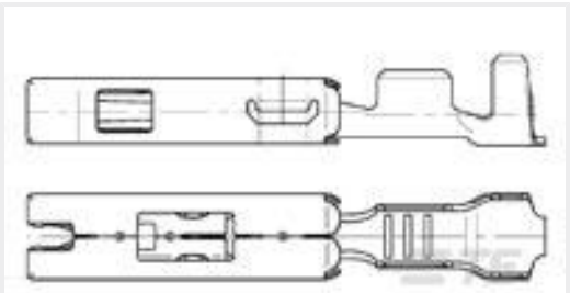
TE 产品编号929025-1 1.5MM SFC
