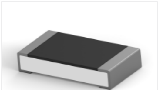
TE 产品编号6-2176388-4 RQ 1206 45R3 0.1% 10PPM 5K RL
