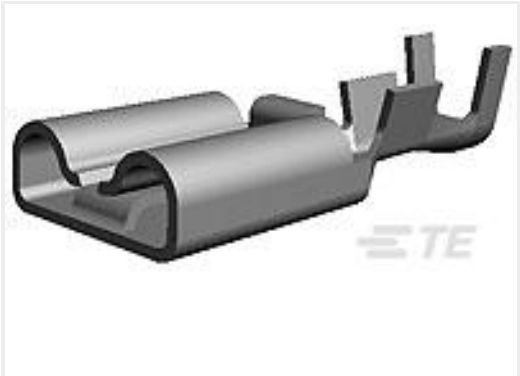
TE 产品编号175020-1 250 PL EX REC. 22-18AWG PTBR
