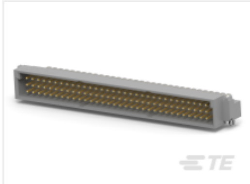
TE 产品编号 5536405-5 ASSY,PIN,EUROCARD,TYPE C,LEAD-
