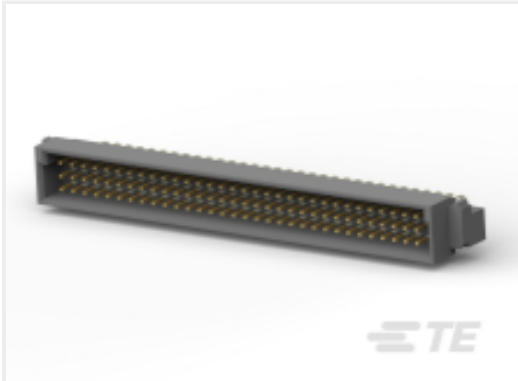
TE 产品编号 5650947-5 ASSY,PIN,EUROCARD,TYPE C,LEAD-
