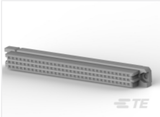
TE 产品编号 5535043-5 ASSY,RECEPTACLE,EUROCARD,TYPE
