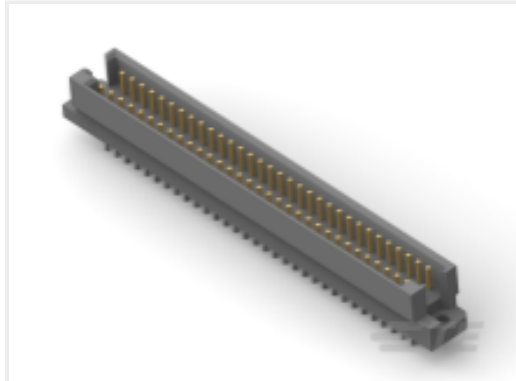
TE 产品编号 650934-5 064 EURO TYPE R PIN ST ASSY
