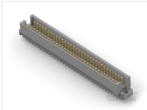
TE 产品编号 650933-5 064 EURO TYPE R PIN ST ASSY
