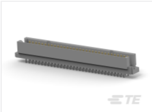
TE 产品编号 5650912-5 ASSY,PIN,EUROCARD,TYPE R,LEAD-FREE,A&C,6
