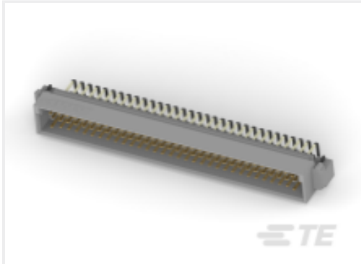
TE 产品编号 536366-5 096 EURO TYPE C PIN MFBL ASSY
