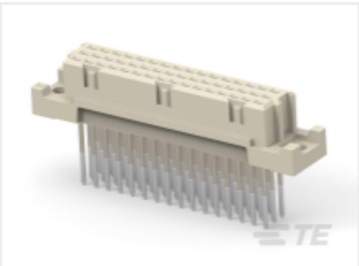
TE 产品编号284172-E STVC/2 48 F ABC VVV 7-00 0606 13,0 * 247
