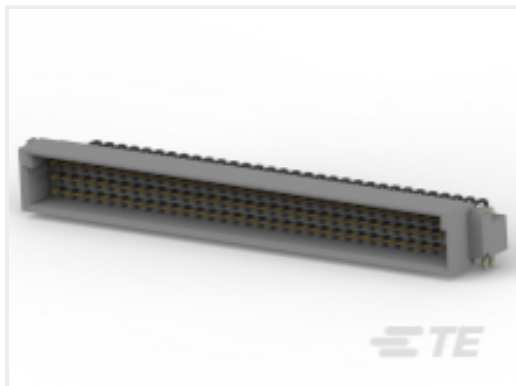
TE 产品编号 5650913-5 ASSY,PIN,EUROCARD,TYPE C,LEAD-OUT
