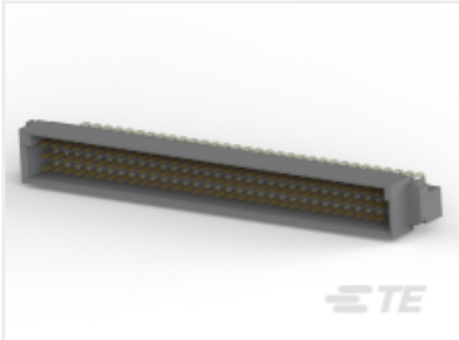
TE 产品编号 5650473-5 ASSY,PIN,EUROCARD,TYPE C,LEAD-OUT
