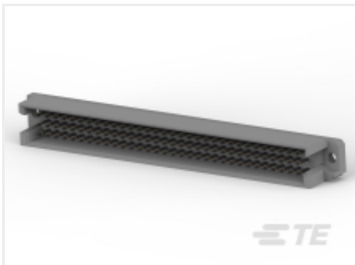
TE 产品编号 5650908-5 ASSY,PIN,EUROCARD,TYPE R,LEAD-OUT
