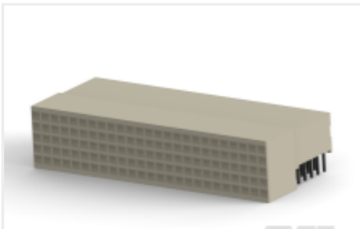
TE 产品编号CAT-472-Z12553 HM 插座连接器：传统背板，共面，2mm
