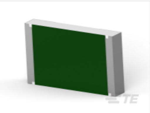
TE 产品编号7-2176401-4 3540 1R8 5%
